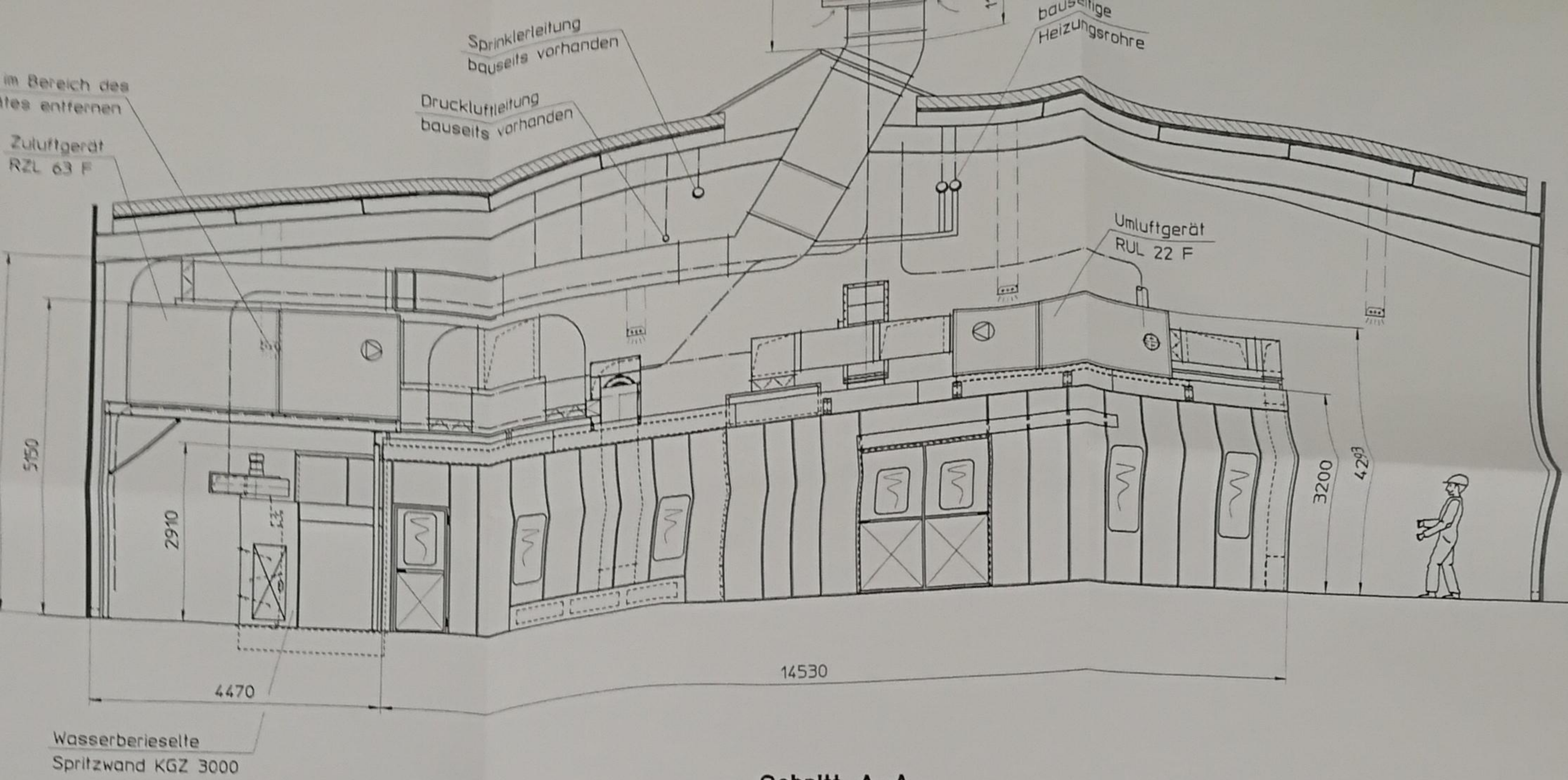
Schnitt A-A
