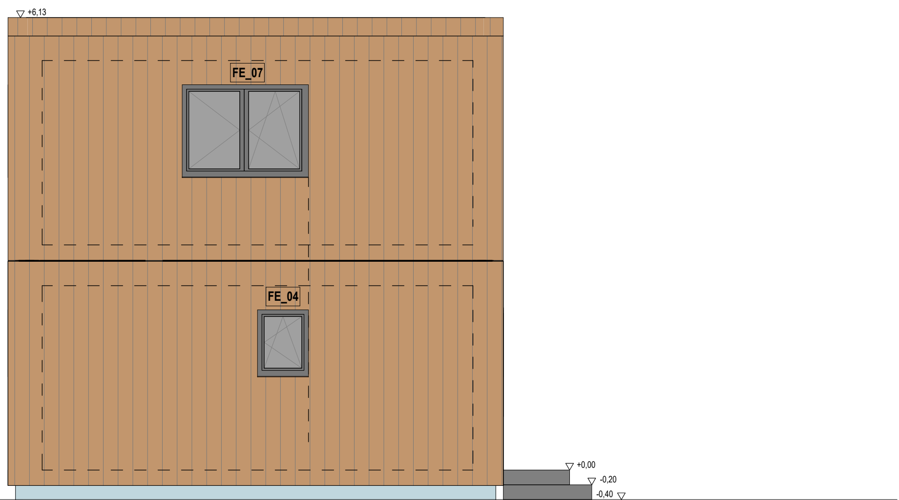
Ansicht West
