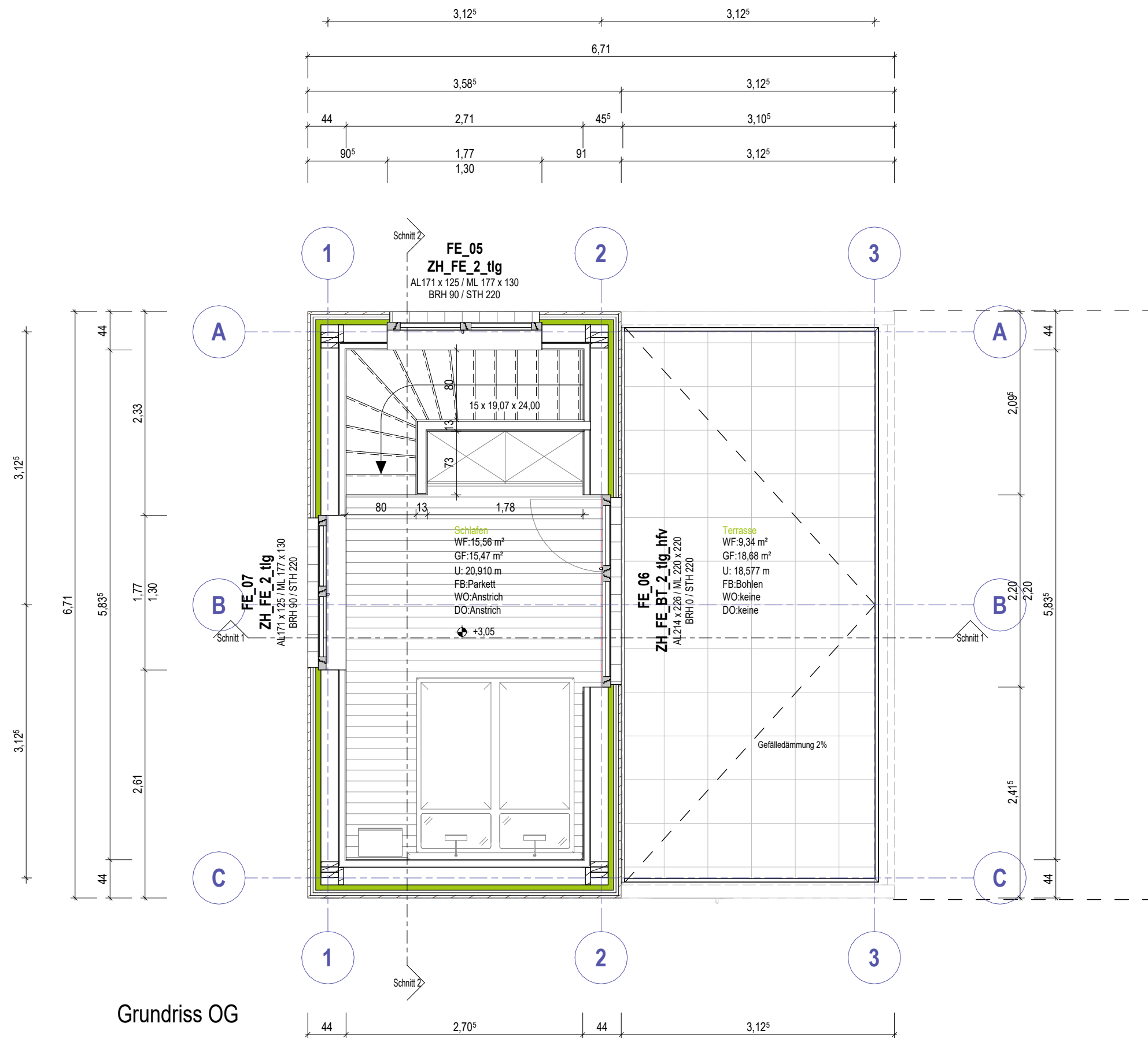
Grundriss OG
